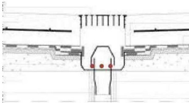
Esquema Sumidero Sifónico. La realización de orificios representada en rojo
